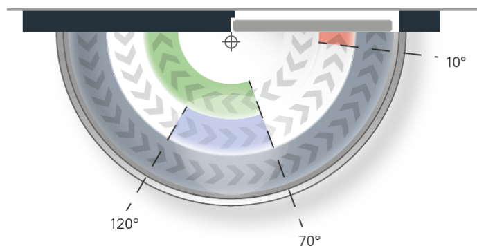
Lukkekræftdiagram ECO Newton TS-62, hængselside
