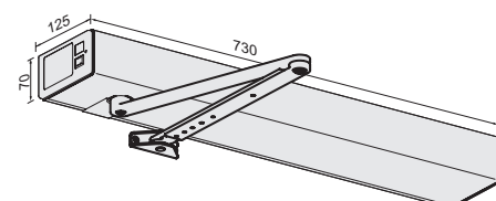
ETS 42 med normal arm
