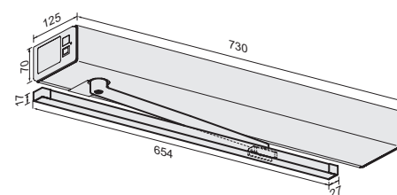
ETS 42 med glideskinne
