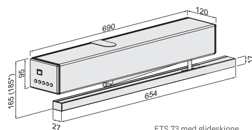
ETS 73 med glideskinne
