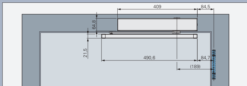
Standard montering, modsat hængselsiden, DIN-R – ECO FTS III
