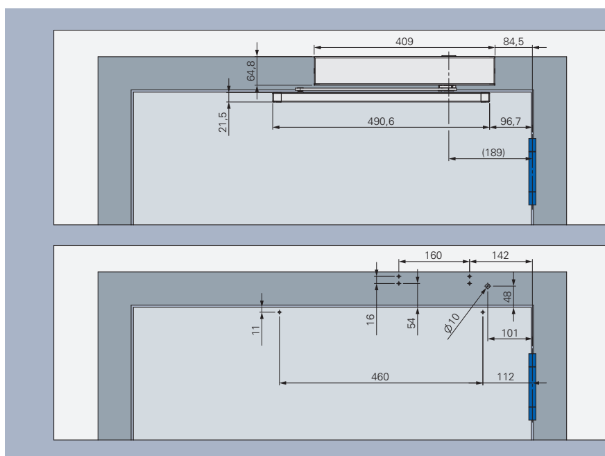
Hovedmontering, hængselsiden, DIN-R – ECO FTS III
