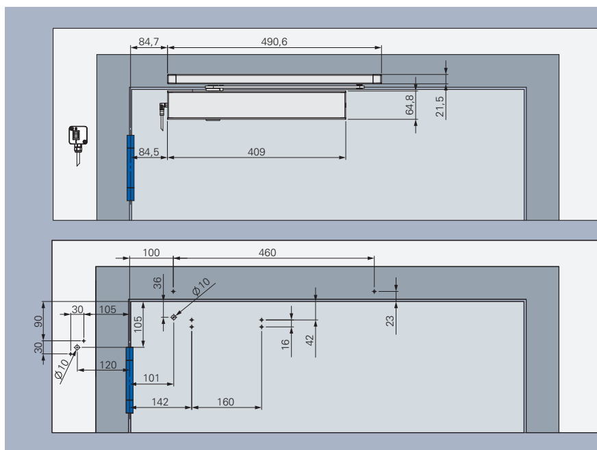
Standard montering, hængselsiden, DIN -L – ECO FTS III
