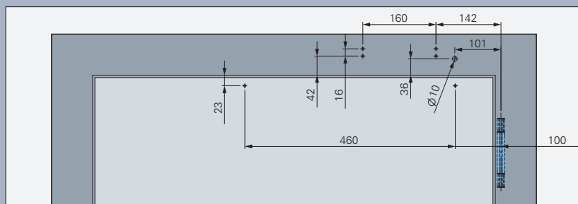
Hoved montering, modsat hængselsiden, DIN-L – ECO FTS III
